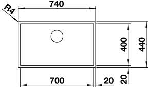
Ausschnitt: 700 x 400 mm Beckentiefe: 185 mm Außenmaß: 740 x 440 mm
