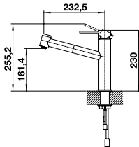
Auslauf 130° schwenkbar mit umstellbaren Schlauchauszug
