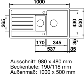
Ablaufgarnitur mit Raumsparrohr, 2 x 3 1/2" Korbventil
