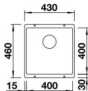
Ausschnitt: 400 x 400 mm Beckentiefe: 190 mm Außenmaß: 430 x 460 mm
