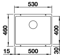
Ausschnitt: 500 x 400 mm Beckentiefe: 190 mm Außenmaß: 530 x 460 mm
