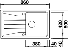
Ausschnitt: 840 x 480 mm Beckentiefe: 190 mm Außenmaß: 860 x 500 mm
