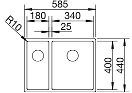
Ausschnitt: 545 x 400 mm Beckentiefe: 130/190 mm Außenmaß: 585 x 440 mm
