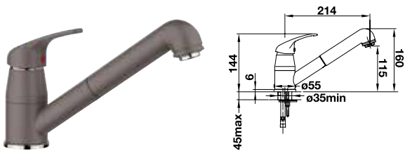
Auslauf 90° schwenkbar mit Schlauchauszug
