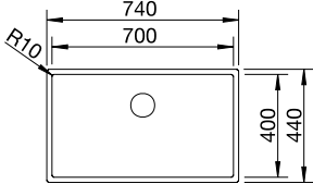
Ausschnitt: 700 x 400 mm Beckentiefe: 190 mm Außenmaß: 740 x 440 mm
