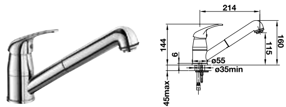
Auslauf 90° schwenkbar mit Schlauchauszug
