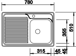
Ausschnitt: 762 x 492 mm Beckentiefe: 195 mm Außenmaß: 780 x 510 mm
