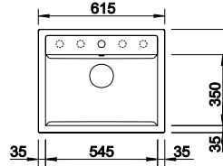
Ausschnitt: 595 x 490 mm Beckentiefe: 190 mm Außenmaß: 615 x 510 mm
