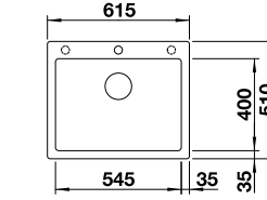
Ausschnitt: 595 x 490 mm Beckentiefe: 220 mm Außenmaß: 615 x 510 mm
