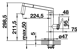
Kaltstart Auslauf 160° schwenkbar mit umstellbarem Schlauchauszug, Metallschlauch
