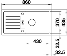
Ausschnitt: 840 x 415 mm Beckentiefe: 180 mm Außenmaß: 860 x 435 mm
