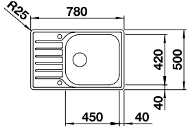
Ausschnitt Einbau von oben: 756 x 476 mm Beckentiefe: 160 mm Außenmaß: 780 x 500 mm
