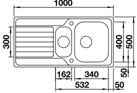
Ausschnitt: 980 x 480 mm Beckentiefe: 190/140 mm Außenmaß: 1000 x 500 mm
