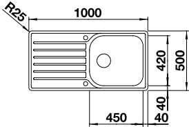
Ausschnitt Einbau von oben: 976 x 476 mm Beckentiefe: 160 mm Außenmaß: 1000 x 500 mm
