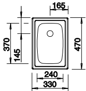
Ausschnitt: 312 x 452 mm Beckentiefe 150 mm Außenmaß 330 x 470 mm
