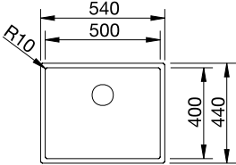
Ausschnittdaten für alle Einbauverfahren finden Sie in unserem Internet-Download Beckentiefe: 190 mm Außenmaß: 540 x 440 mm
