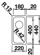
Ausschnitt: 180 x 400 mm Beckentiefe: 130 mm Außenmaß: 220 x 440 mm
