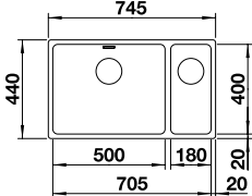
Ausschnitt: 705 x 400 mm Beckentiefe: 130/190mm Außenmaß: 745 x 440 mm
