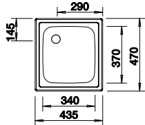
Ausschnitt: 417 x 452 mm Beckentiefe 150 mm Außenmaß 435 x 470 mm
