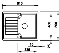
Ausschnitt: 595 x 480 mm Beckentiefe: 190 mm Außenmaß: 615 x 500 mm
