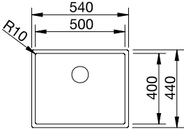
Ausschnitt: 500 x 400 mm Beckentiefe: 190 mm Außenmaß: 540 x 440 mm
