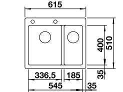
Ausschnitt: 595 x 490 mm Beckentiefe: 220 mm Außenmaß: 600 x 510 mm
