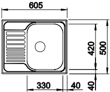
Ausschnitt: 587 x 482 mm Beckentiefe: 160 mm Außenmaß: 605 x 500 mm
